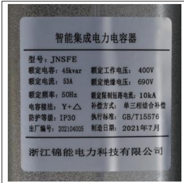
铭牌
